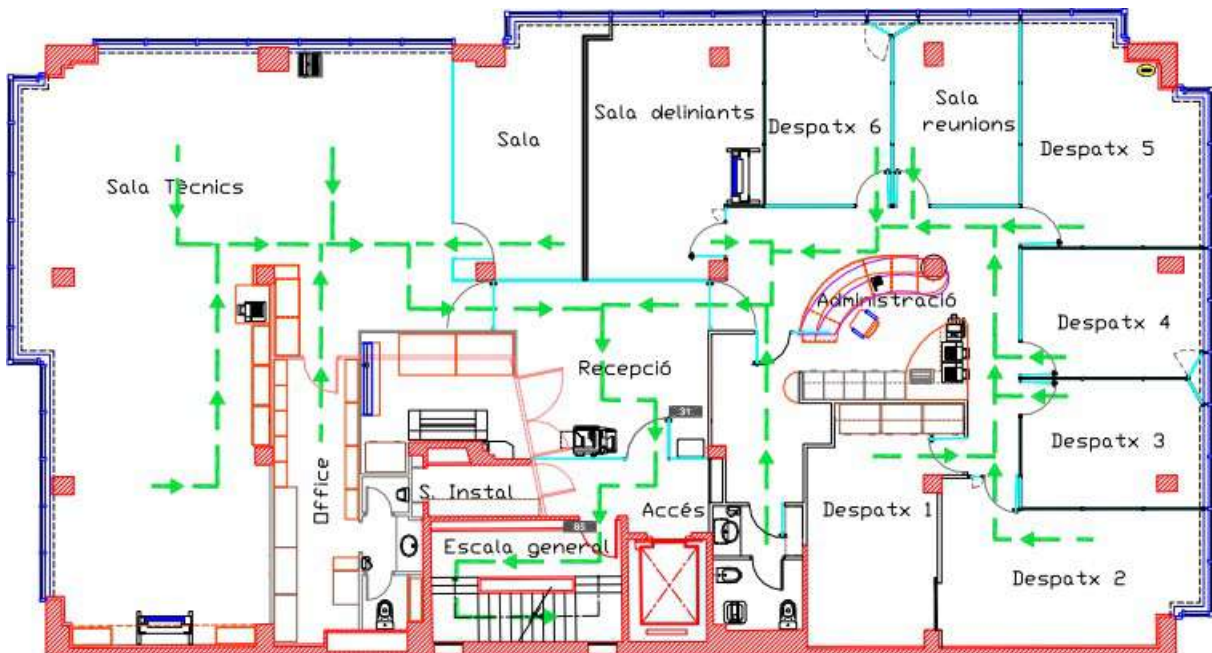
PLANTA QUARTA
