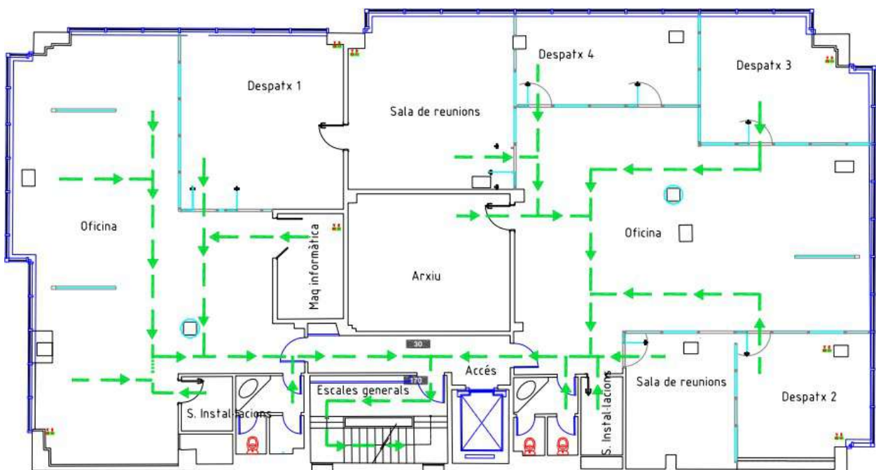
PLANTA PRIMERA
