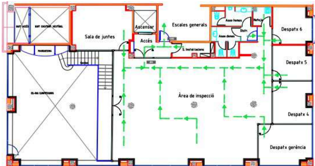
PLANTA ALTELL
