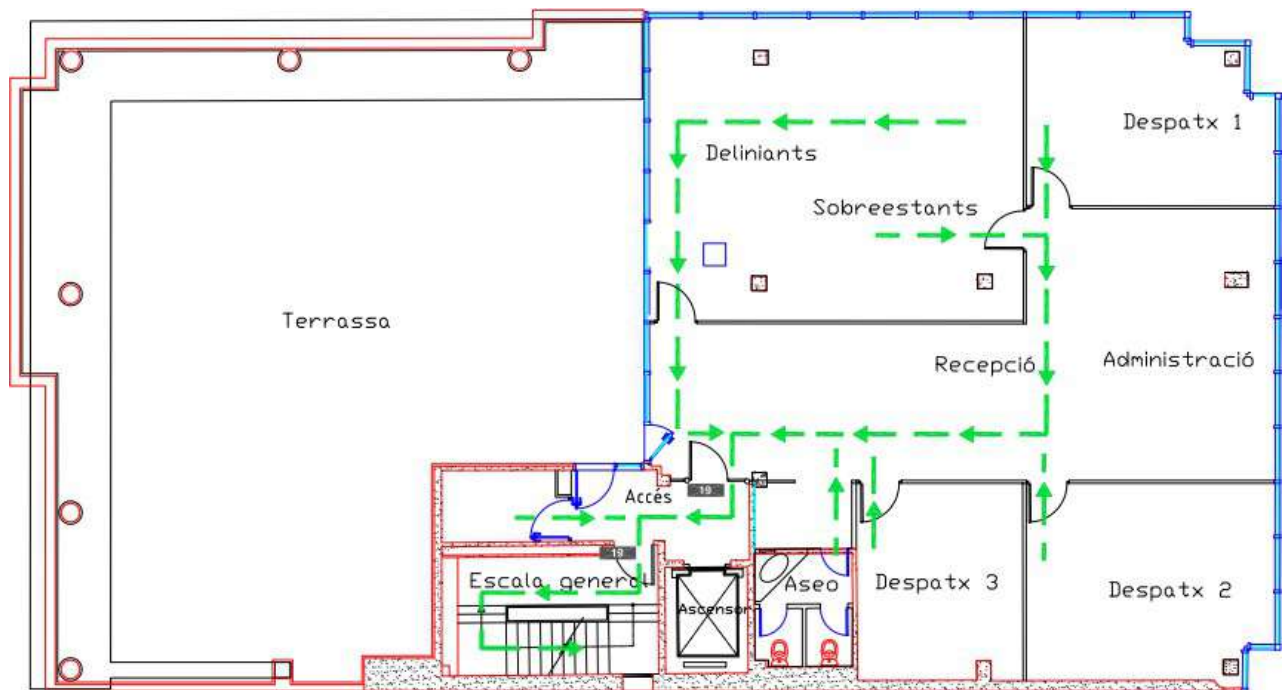
PLANTA SISENA
